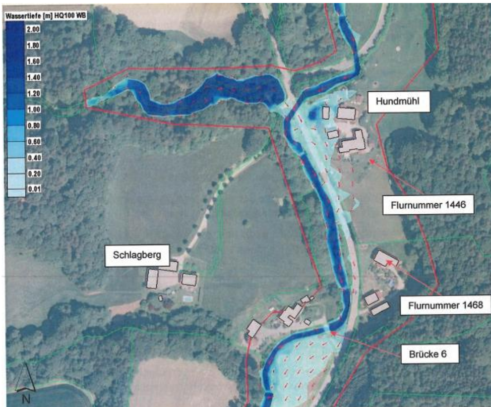
Abbildung 6.1: Gewässerabschnitt Weitbach Ortsteil Hundmühl / Kreisstraße AÖ8, HQ 100 WB
